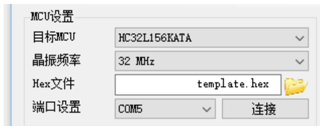
图 12 MCU 设置
