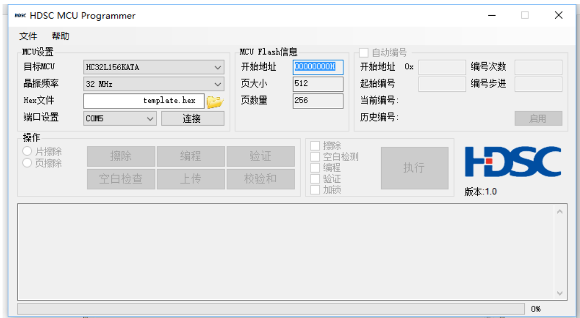
图 8 MCU 设置
