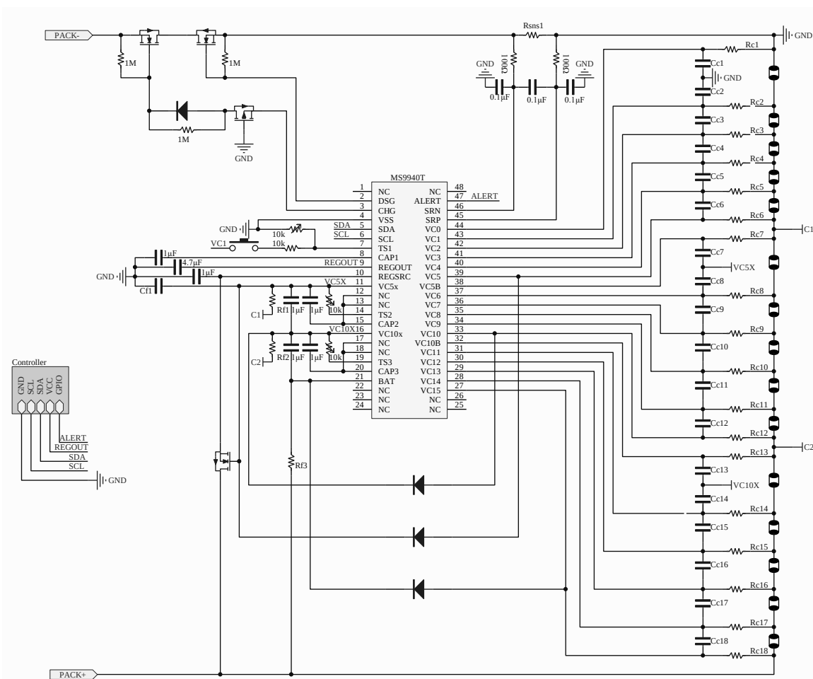
MS9940T 典型应用图
