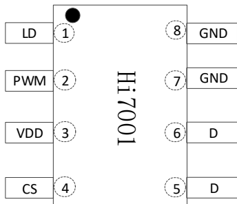
图 5.1 Hi7001 管脚图
