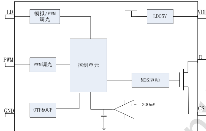
图 7.1 结构框图
