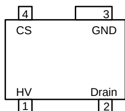
SOT33-4
