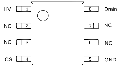
ESOP-8
