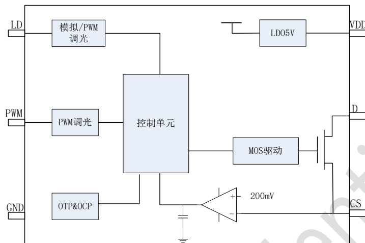
图 7.1 结构框图
