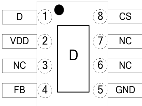
(EP 管脚为底部散热盘) Hi9103B 管脚图
