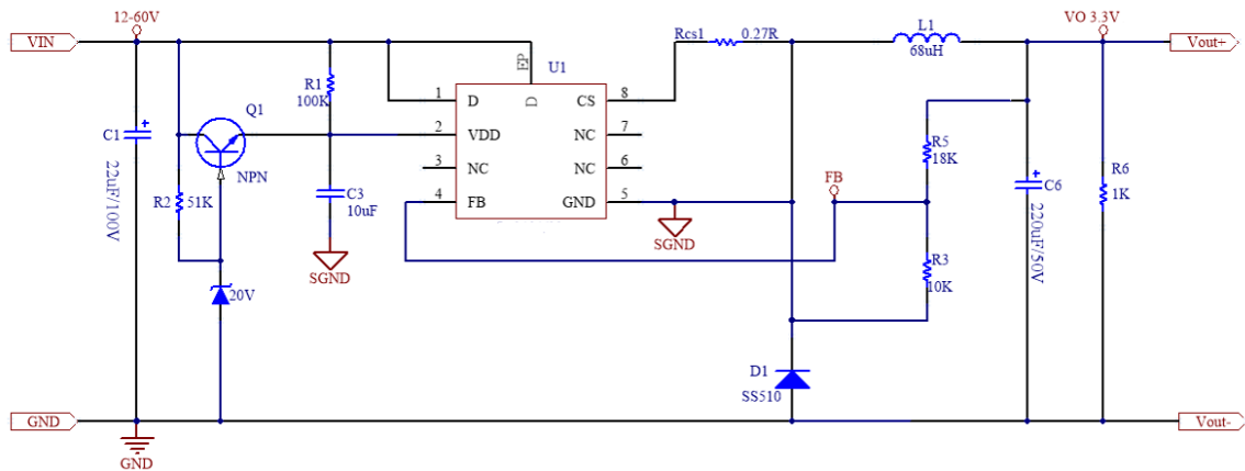
12~60V 输入----3.3V/0.8A 输出应用图
