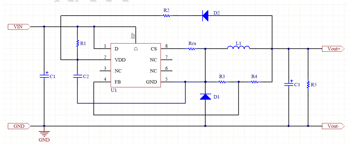
典型应用电路
