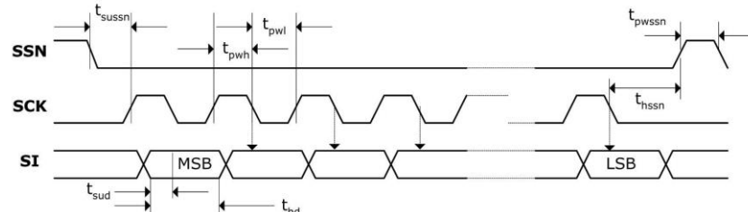
图 1. SPI 写时序
