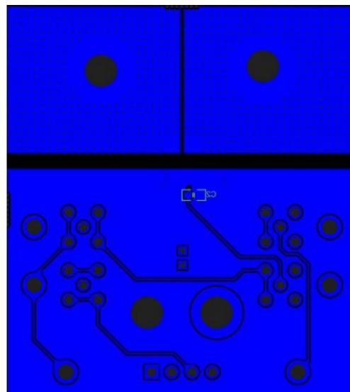
图 8.Demo 板反面
