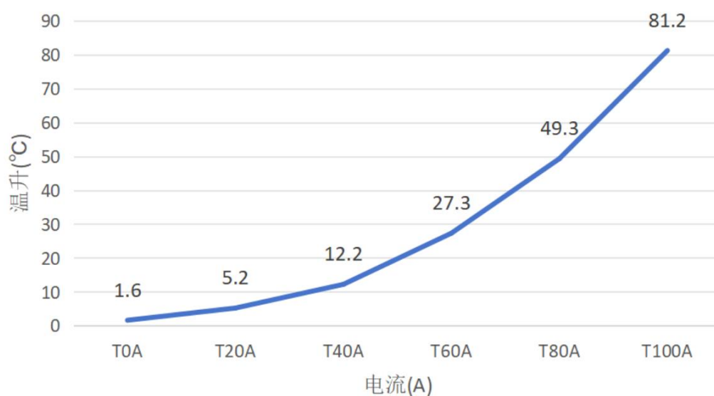
图 6.温升曲线图
