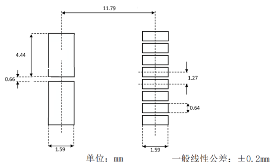
图 10. 推荐焊盘尺寸
