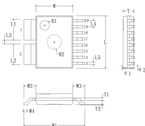
图 9. SOIC-10 封装
