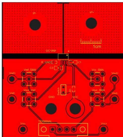
图 7.Demo 板正面
