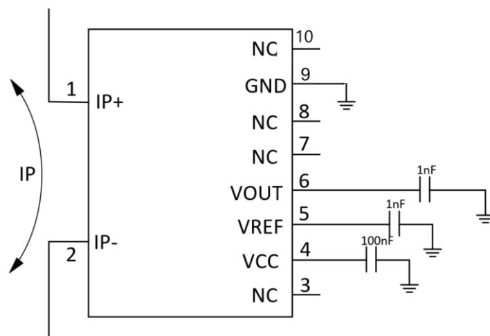
图 3. 应用电路
