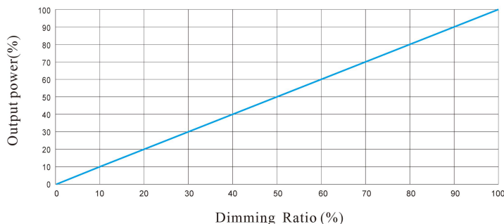
输出功率Vs. 调光信号
