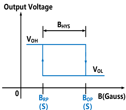
TO-92S 输出状态
